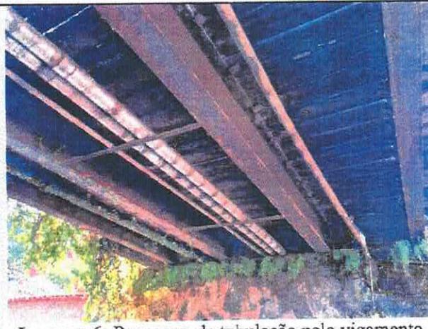
Imagem 6: Passagem de tubulação pelo vigamento
