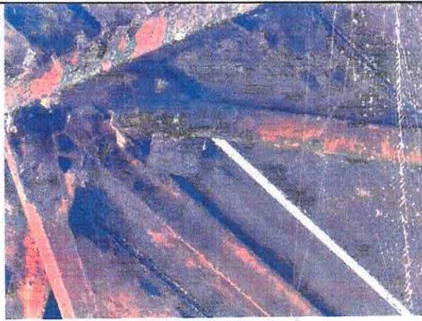
Imagem 6: Degradação de vigamento
